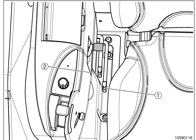
①作業機電源 (20Aヒューズ)
