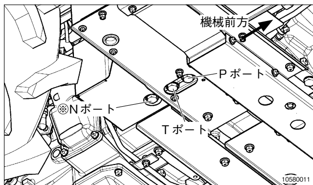
※六角穴付プラグ (Rc1/4) をネジ込む
